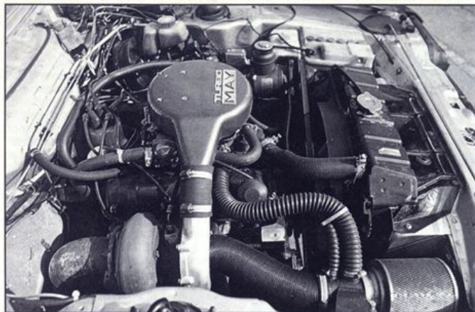
Das May-Turbo-System mit Ladereinheit von KKK (links vorne)
